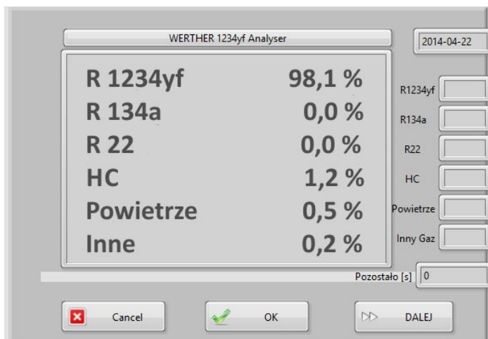
Fot. 5. Pulpit sterowniczy identyfikatora – stacja obsługowa Werther
