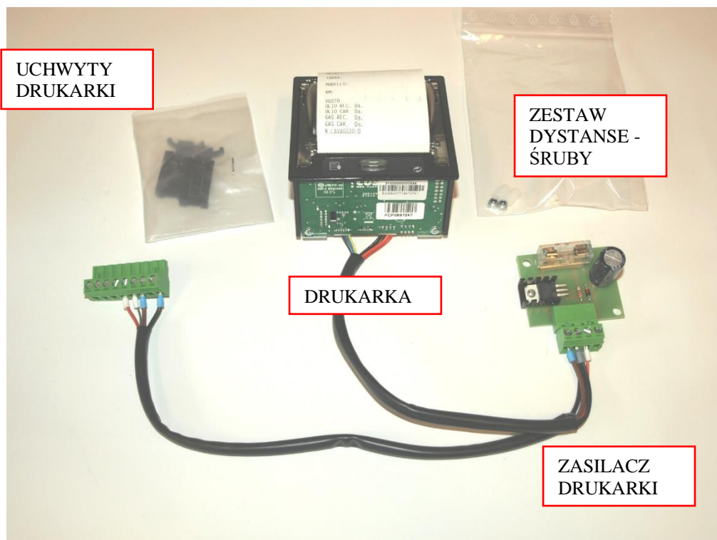
Rys. Zestaw instalacyjny drukarki
